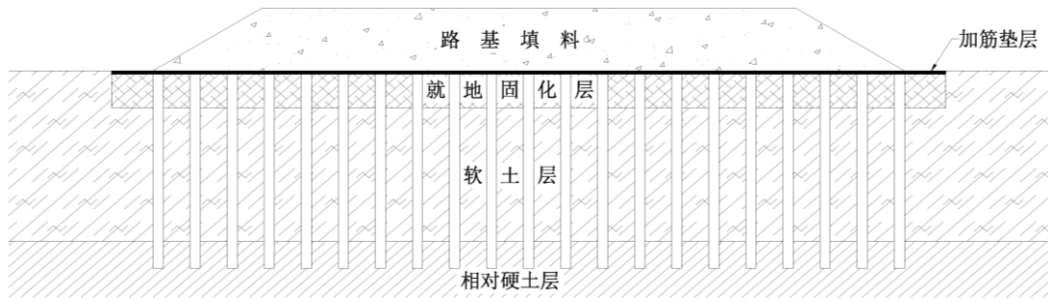
d) 不设桩帽柔性桩复合地基（打穿软土层）
