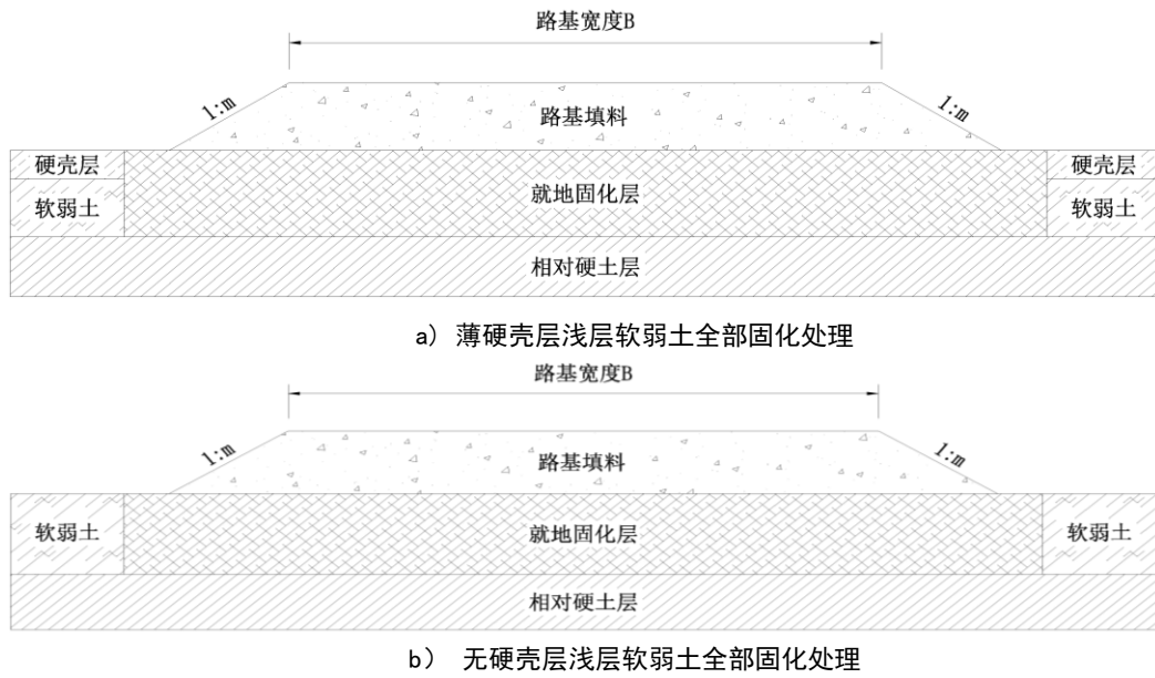
图3 浅层软弱土全部固化处理示意图
