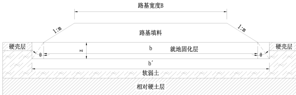
图10 就地固化硬壳层宽度要求示意图
