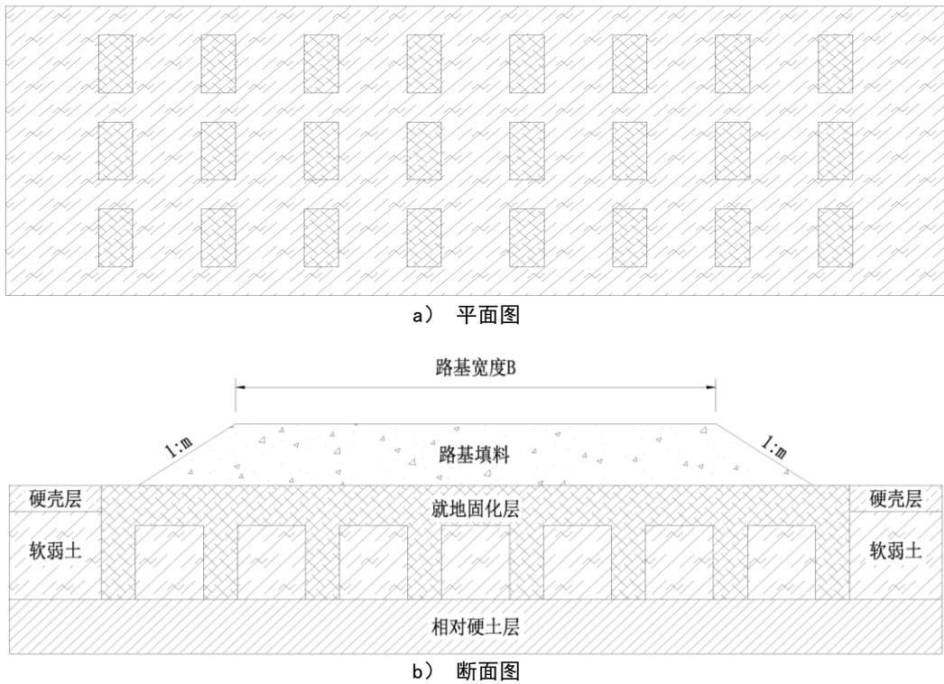
图6 浅层软弱土部分固化处理（全断面固化组合点式固化）示意图
