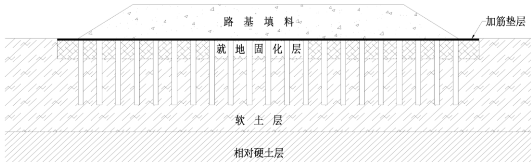
e) 不设桩帽柔性桩复合地基（未打穿软土层）
