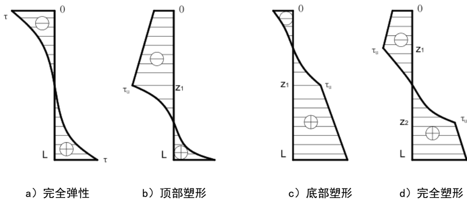
图 D.6 桩侧摩阻力沿桩身分布图
