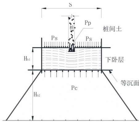
图 D.7 下卧层受力计算模型
